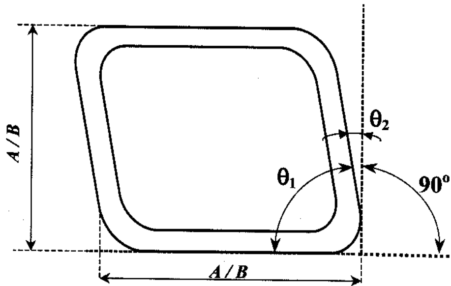
Рис. 6 Отклонение прямоугольности сторон труб квадратного, прямоугольного и полуовального сечений
